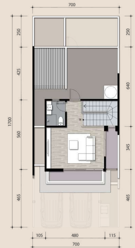
3 RD F
